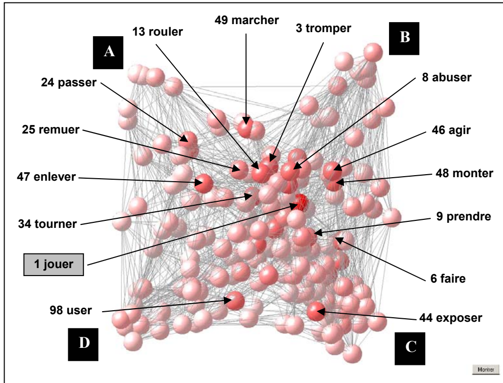
Figure 25 La proxémie de « jouer » pour \lambda=6 dans V_{6,V,200}
