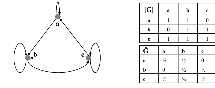
Figure 1 un graphe G réflexif et \hat{G} sa matrice Markovienne
