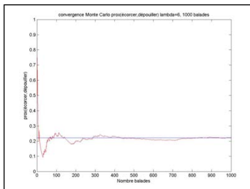
Figure 26 Convergence vers [\hat{G}^6]_{\text{écorder,dépouiller}} Méthode Monte Carlo : \lambda=6 , q=1000
